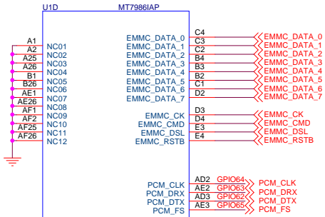
02:eMMC
