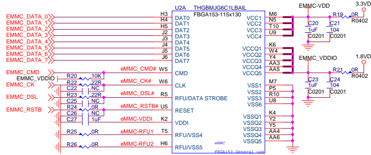
02:eMMC
